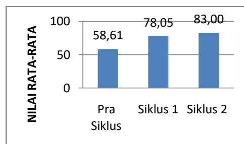
Grafik 4.5 Rata-Rata Hasil Evaluasi Prasiklus, Siklus 1, dan Siklus 2
